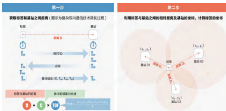
图 3-5 UWB TOF 算法
