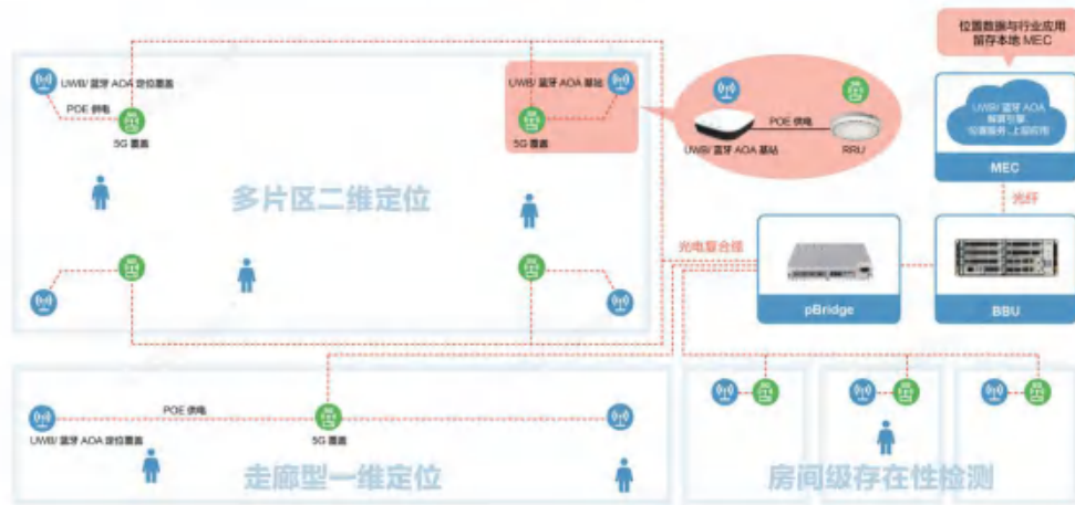
图 5-2 系统整体部署架构
