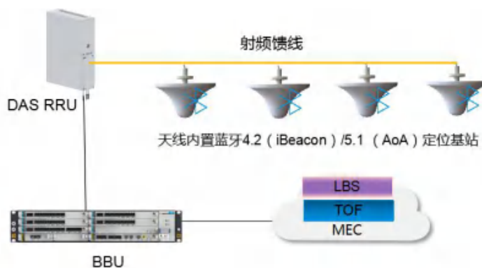
图 4-6 5G+传统蓝牙组网架构图
