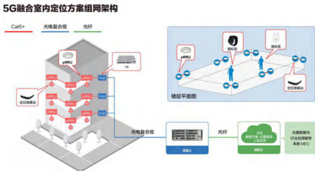
图 4-5 5G 融合 UWB/蓝牙 AOA 组网架构
