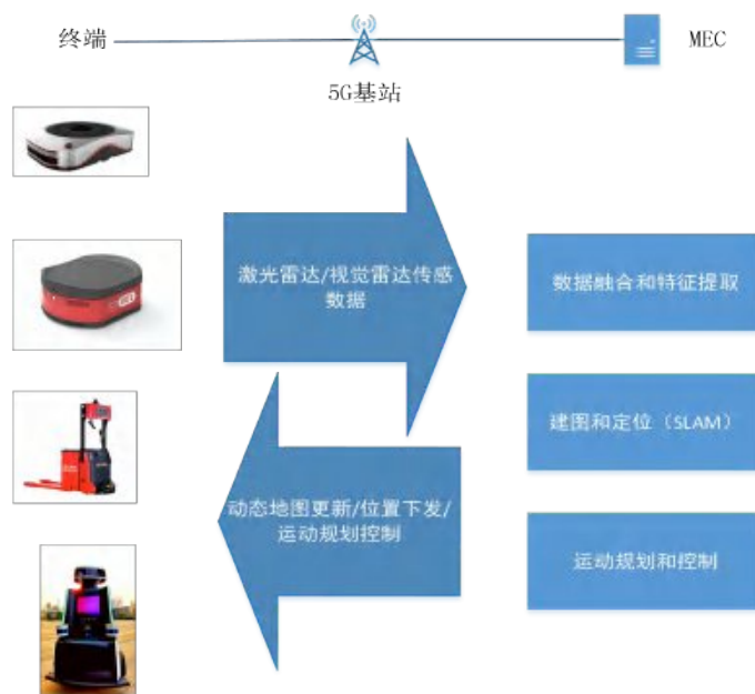
图 4-8 5G+SLAM 定位方案
