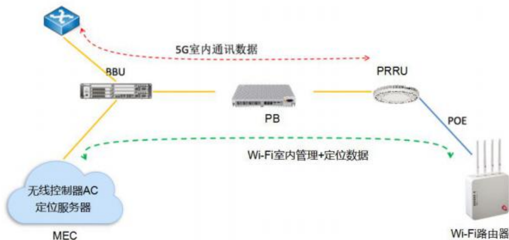
图 4-75G+Wi-Fi 组网架构图
