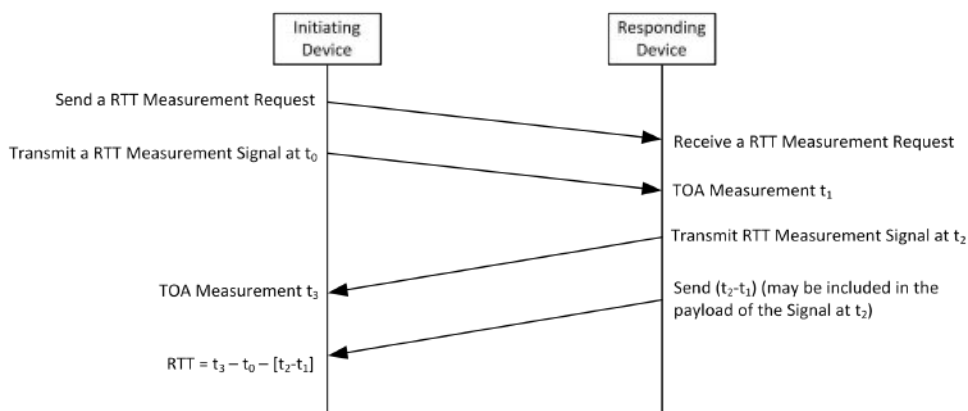
图 4- 4 RTT定位交互示意图
