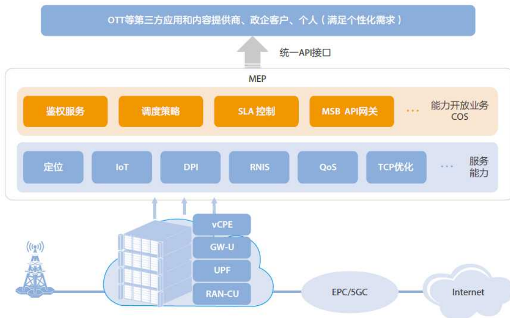
图 3-3 MEC 部署图
